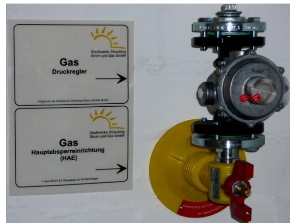
Bild 2: Hauptabsperreinrichtung mit Druckregler im Keller
