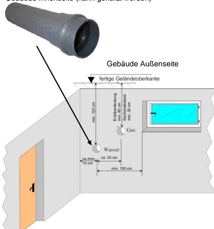
Bild 1: Mauerdurchführung / Futterrohr
